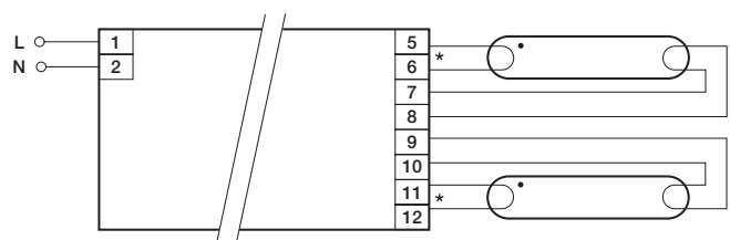
EcoTronic 2/18–2/58W
